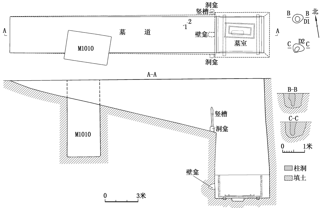
图三 M1011 平面、剖面、剖视图
