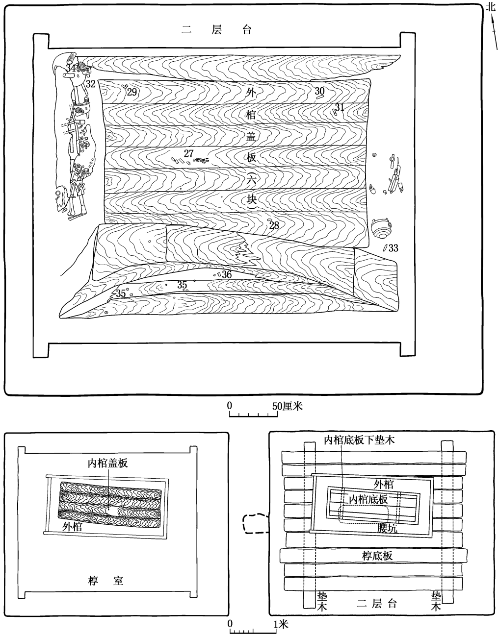
图五 葬具盖板及底板平面图
