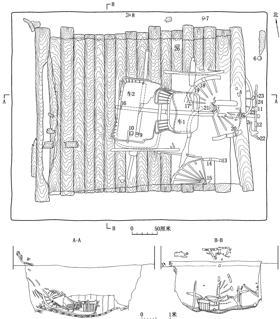
图四 椁盖板及随葬车平面、剖视图
